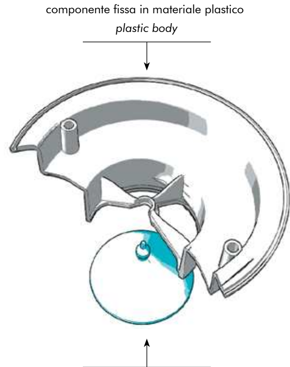
valvola di scarico in silicone ad apertura e chiusura automatica exhaust automatic silicon valve
