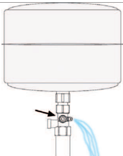
Scaricare il liquido rimanente nel vaso tramite il ribunetto e procedere con la rimozione del vaso. Drain remaining water in tank by opening tap, then remove tank for service or replace it.
