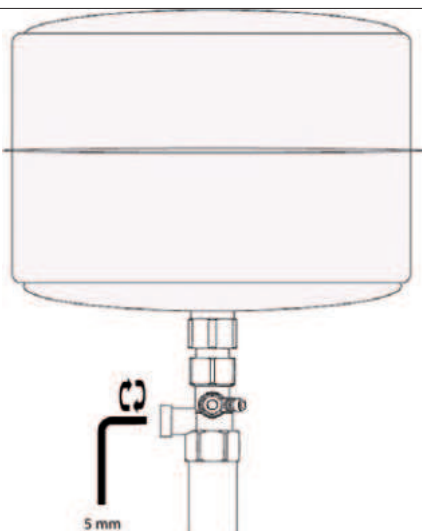
Isolare il vaso chiudendo la valvola con una chiave Ø 5mm Close tank valve with a 5mm allen wrench
