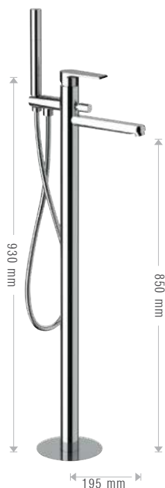
21A/AT € 950,00 Miscelatore monocomando vasca da pavimento. Single lever bath mixer floor-mounting.
