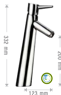
397/SN € 210,00 Miscelatore monocomando lavabo alto, senza scarico. Single lever basin mixer high neck, without waste.
