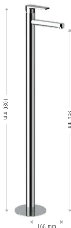
385/AT € 850,00 Miscelatore monocomando lavabo da terra senza scarico. Single lever basin mixer for floor-mounting without waste.
