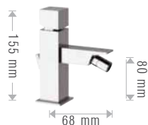
493/CB € 210,00 Miscelatore monocomando bidet. Single lever bidet mixer.
