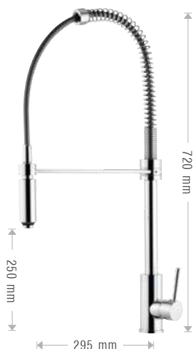
57A/HR € 410,00 Miscelatore monocomando lavello a molla con doccetta estraibile a 2 funzioni. Single-lever sink mixer with spring spout and 2 functions pull-out hand shower.
