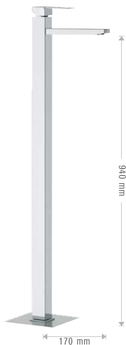
385/PA € 1.000,00 Miscelatore monocomando lavabo da terra senza scarico. Single-lever basin mixer floor-mounting without waste.
