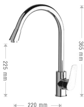
506/ES € 135,00 Miscelatore monocomando lavello con bocca girevole. Single lever sink mixer with swivel spout.
