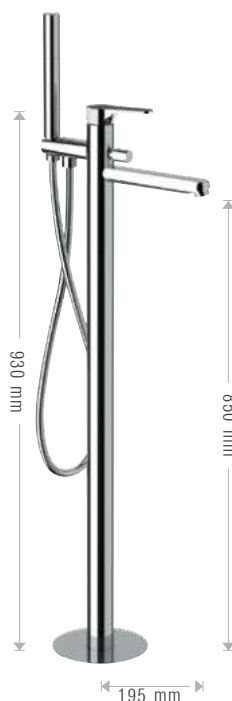
21A/SF € 950,00 Miscelatore monocomando vasca da pavimento. Single lever bath mixer floor-mounting.
