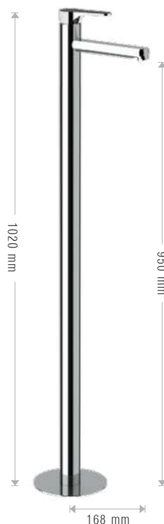
385/SF € 850,00 Miscelatore monocomando lavabo da terra senza scarico. Single lever basin mixer for floor-mounting without waste.
