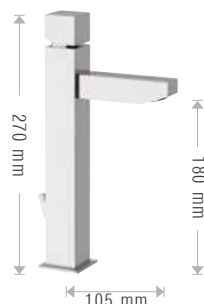
397/CB € 225,00 Miscelatore monocomando lavabo alto senza scarico. Single lever basin mixer high neck, without pop-up waste.
