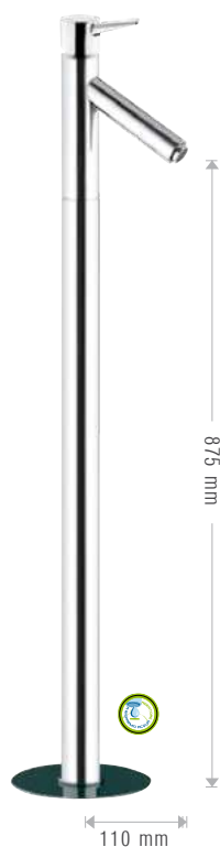
385/SN € 900,00 Miscelatore monocomando lavabo da terra senza scarico. Single lever basin mixer for floor-mounting without waste.
